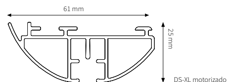
DS-XL motorizado
